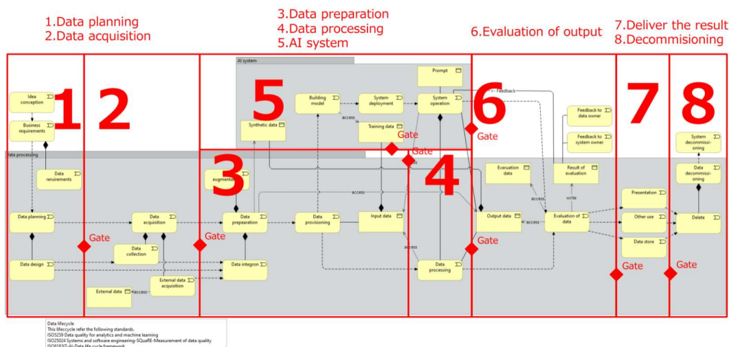
図 3-7 AI システムも含めたデータライフサイクル
